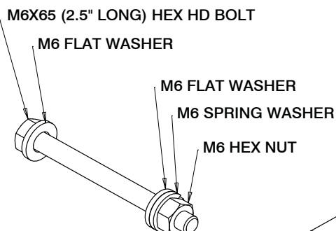
M6 BOLT ASSEMBLY QTY: 2
